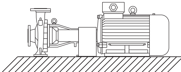
Рисунок.4. горизонтальное расположение насоса на фундаменте.
