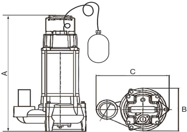
Габаритные размеры
