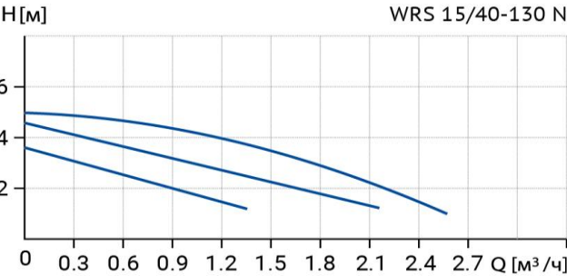
Диаграмма характеристик
