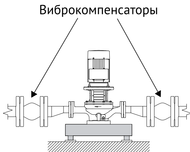
Рис. 8. Насос TG с виброкомпенсаторами большего диаметра.
